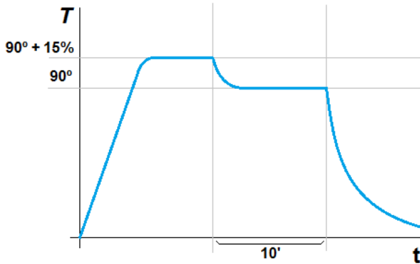
Figura 8: Temperatura horno.
