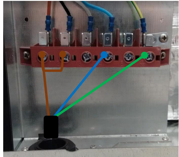
Figura 9: Conexión monofásica media potencia
