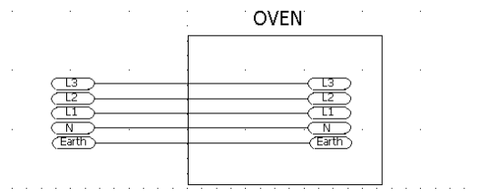
Figura 4: Conexión trifásica 400V 3L+N.
