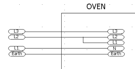
Figura 6: Conexión trifásica 230V 3L.
