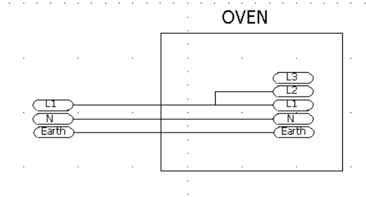
Figura 8: Conexión monofásica media potencia
