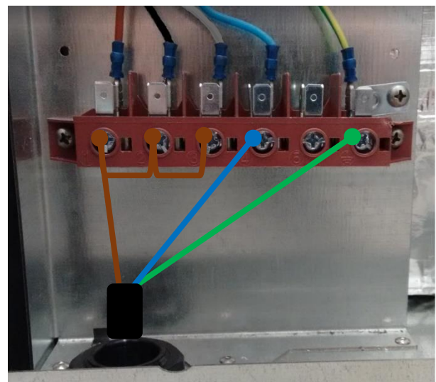
Figura 11: Conexión monofásica plena potencia.
