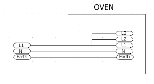
Figura 10: Conexión monofásica plena potencia.
